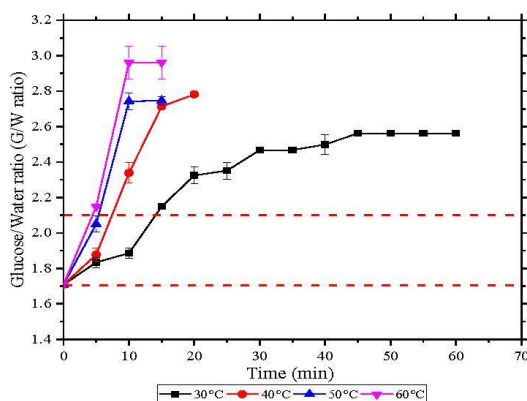
192 ภาพที่ 4 กราฟแสดงความสัมพันธ์ระหว่างสัดส่วนน้ำตาลกลูโคสต่อน้ำ (G/W ratio) กับเวลา ด้วย
