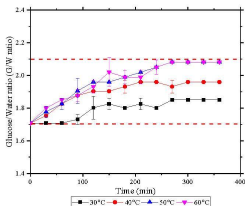
219 220 ภาพที่ 6 กราฟแสดงความสัมพันธ์ระหว่างสัดส่วนน้ำตาลกลูโคสต่อน้ำ (G/W ratio) กับเวลา ด้วยเครื่องอบแบบลมร้อน ที่ 221 อุณหภูมิ 30, 40, 50 และ 60 องศาเซลเซียส
